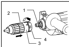
1. 主轴 2. 快换式钻机夹盘 3. 转换套指示线 4. 转换套
