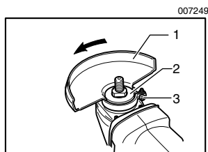
1. 砂轮罩 2. 轴承箱 3. 螺丝
