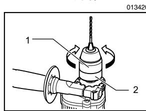
1. 套筒 2. 挡圈
